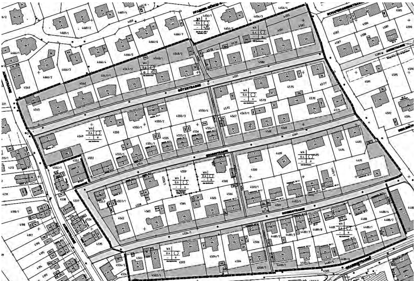
Lageplan zur 4. Änderung des Bebauungsplans "Beinlen", Stand 11.3.2015
